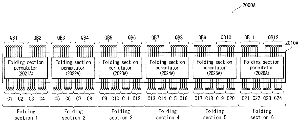
FIG. 32
