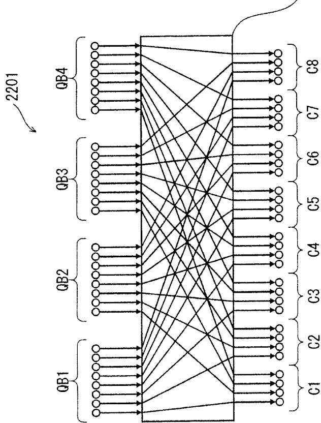
FIG. 22A
