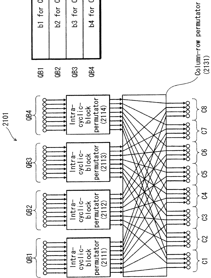
FIG. 21A
