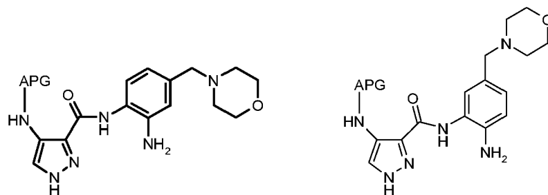
(XXVIIa)
