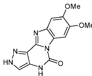
(XXXIVa)
