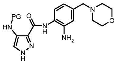
(XXVII)
