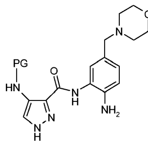
(XXVIII)
