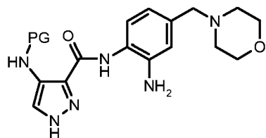
(XXVII)
