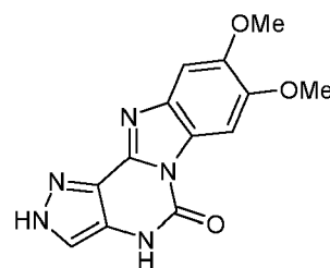
(XXXIVa)
