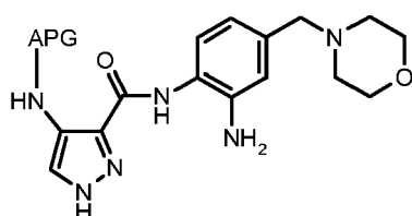
(XXVIIa)
