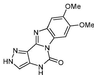
(XXXIVa)
