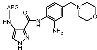
(XXVIIa)
