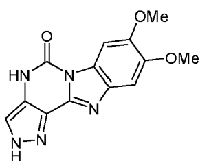
(XXXIV)
