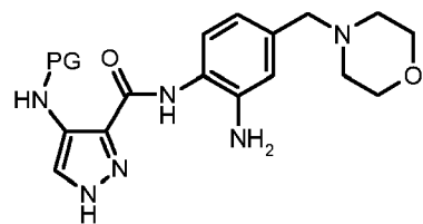
(XXVII)
