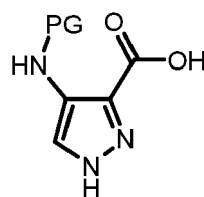
(XXIX)
