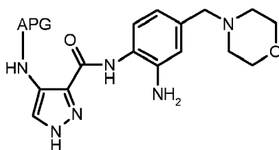
(XXVIIa)
