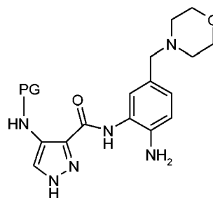
(XXVIII)
