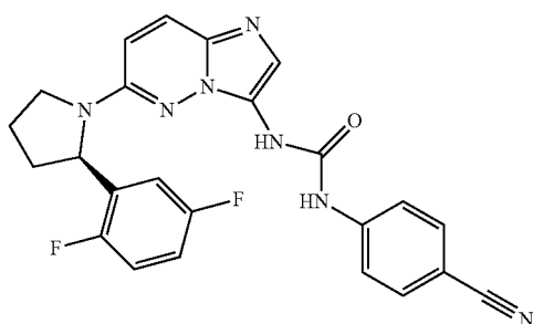
(R)-1-(4-cyanophenyl)-3-(6-(2-(2,5-difluorophenyl)pyrrolidin-1-yl)imidazo[1,2-b]pyridazin-3-yl)urea
