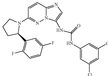
(R)-1-(3,5-dichlorophenyl)-3-(6-(2-(2,5-difluorophenyl)pyrrolidin-1-yl)imidazo[1,2-b]pyridazin-3-yl)urea
