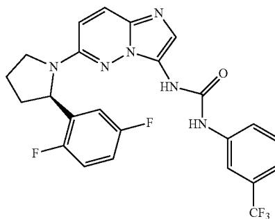
(R)-1-(6-(2-(2,5-difluorophenyl)pyrrolidin-1-yl)imidazo[1,2-b]pyridazin-3-yl)-3-(3-(trifluoromethyl)phenyl)urea
