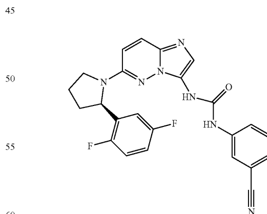
(R)-1-(3-cyanophenyl)-3-(6-(2-(2,5-difluorophenyl)pyrrolidin-1-yl)imidazo[1,2-b]pyridazin-3-yl)urea
