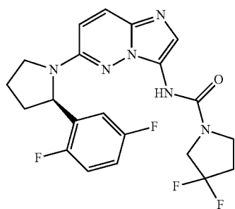
(R)-N-(6-(2-(2,5-difluorophenyl)pyrrolidin-1-yl)imidazo[1,2-b]pyridazin-3-yl)-3,3-difluoropyrrolidine-1-carboxamide
