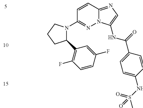
(R)—N-(6-(2-(2,5-difluorophenyl)pyrrolidin-1-yl)imidazo[1,2-b]pyridazin-3-yl)-4-(methylsulfonylamido)benzamide
