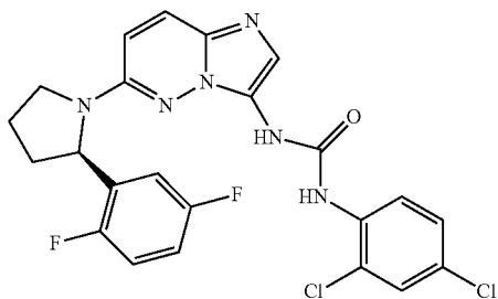
(R)-1-(2,4-dichlorophenyl)-3-(6-(2-(2,5-difluorophenyl)pyrrolidin-1-yl)imidazo[1,2-b]pyridazin-3-yl)urea
