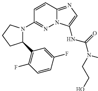
(R)-3-(6-(2-(2,5-difluorophenyl)pyrrolidin-1-yl)imidazo[1,2-b]pyridazin-3-yl)-1-(2-hydroxyethyl)-1-methylurea
