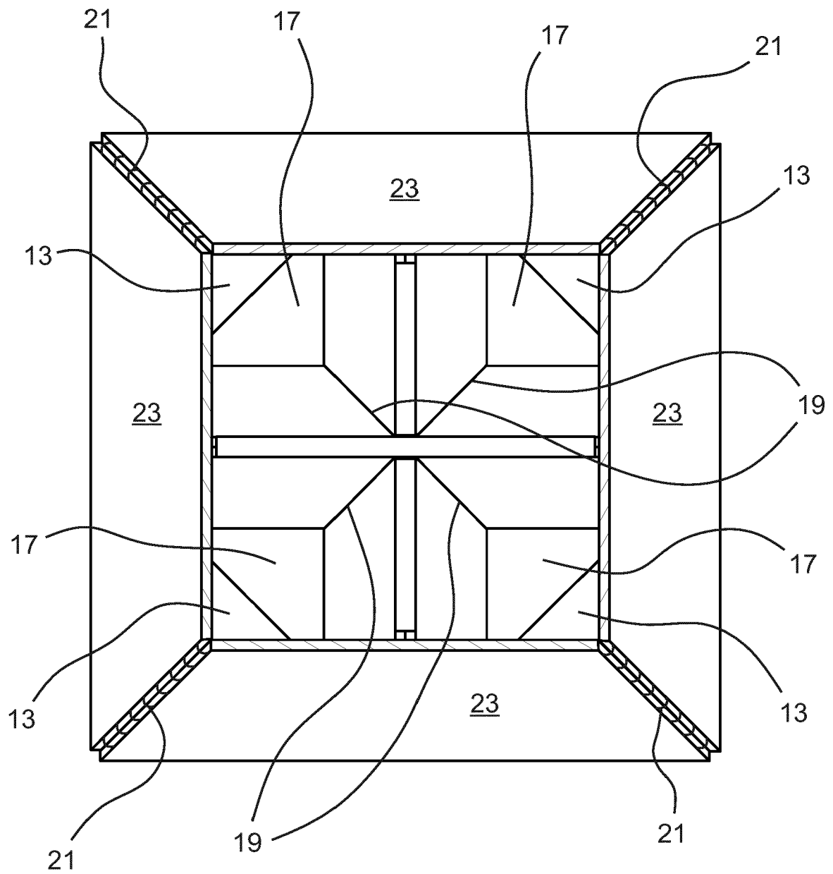
Section A-A
