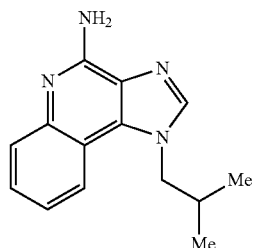
Imiquimod
