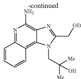
Resiquimod
