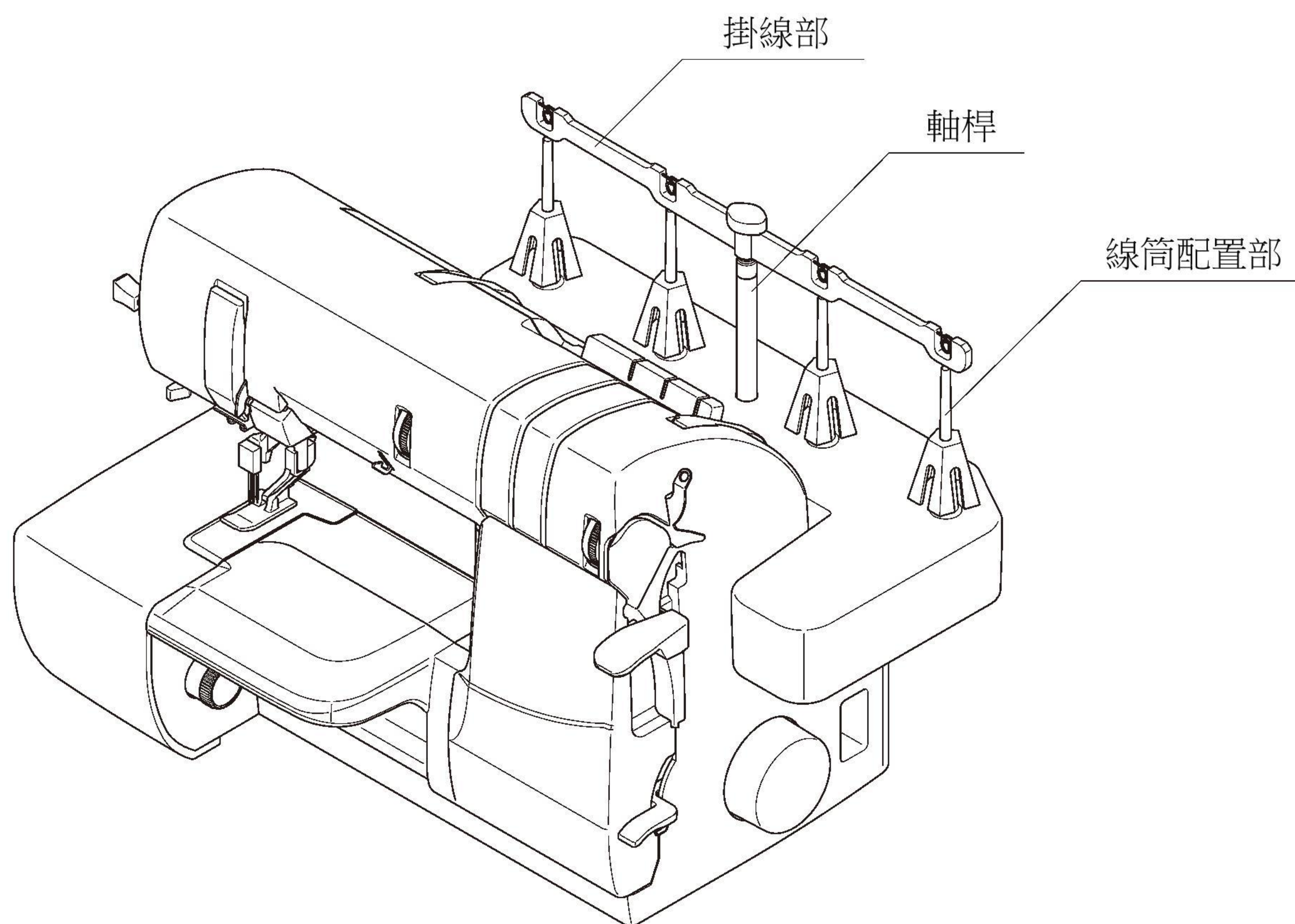
【收縮軸桿狀態之標示各部名稱之參考立體圖】
