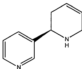
R-(+)-anatabine
