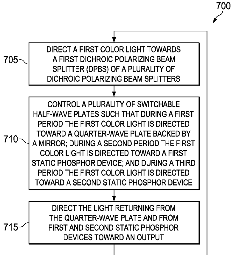
FIG. 7A
