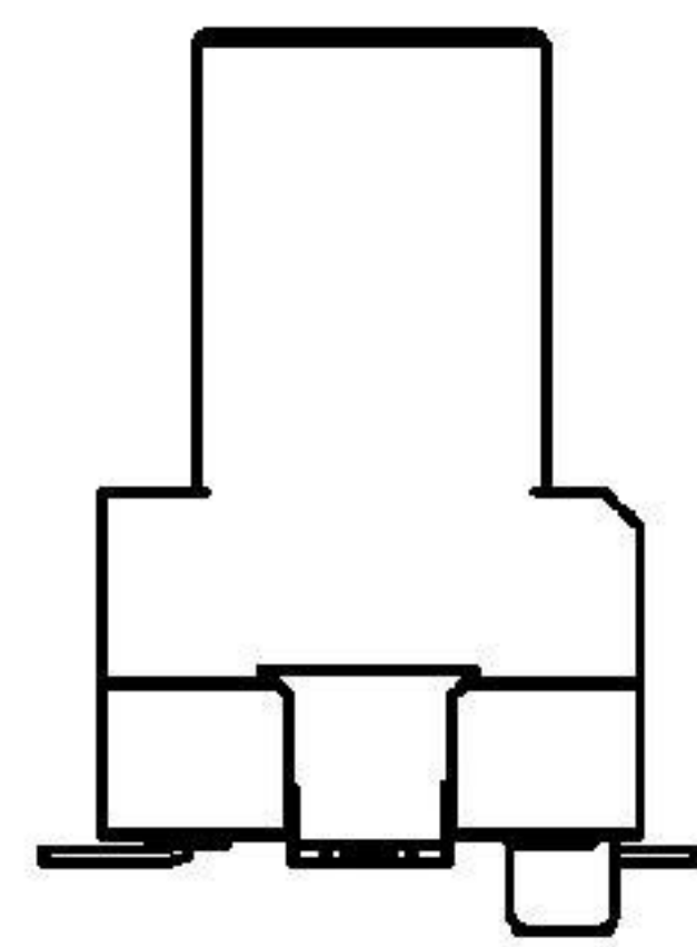
【左側視圖】
