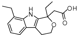
Etodolac
