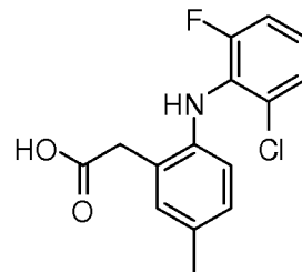
Lumiracoxib
