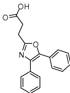
Oxaprozin
