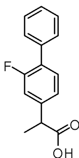
Flurbiprofen
