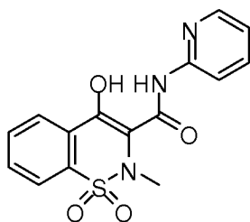
Piroxicam
