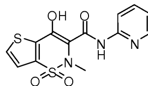
Tenoxicam
