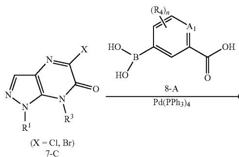
Scheme 2 (Method B)
