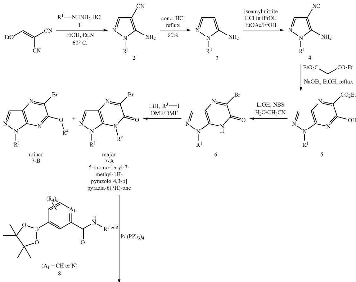
Scheme 1 (Method A)
