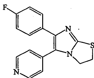
P1 SK&F 86002
