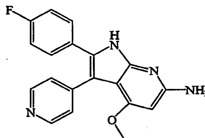
P5 RWJ 68354
