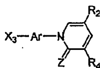
Genus VI
