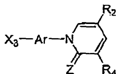
Genus VI
