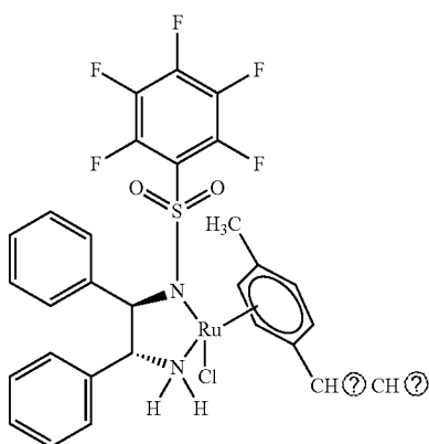
RuCl(FsDPEN)(p-cymene)
