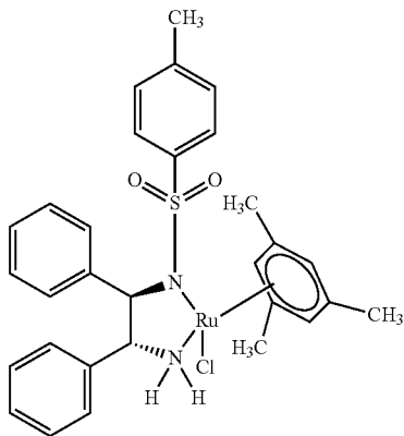
RuCl(TsDPEN)(mesitylene)
