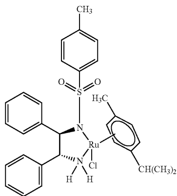
RuCl(TsDPEN)(p-cymene)
