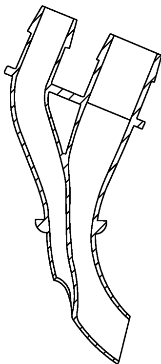
SECTION A-A
