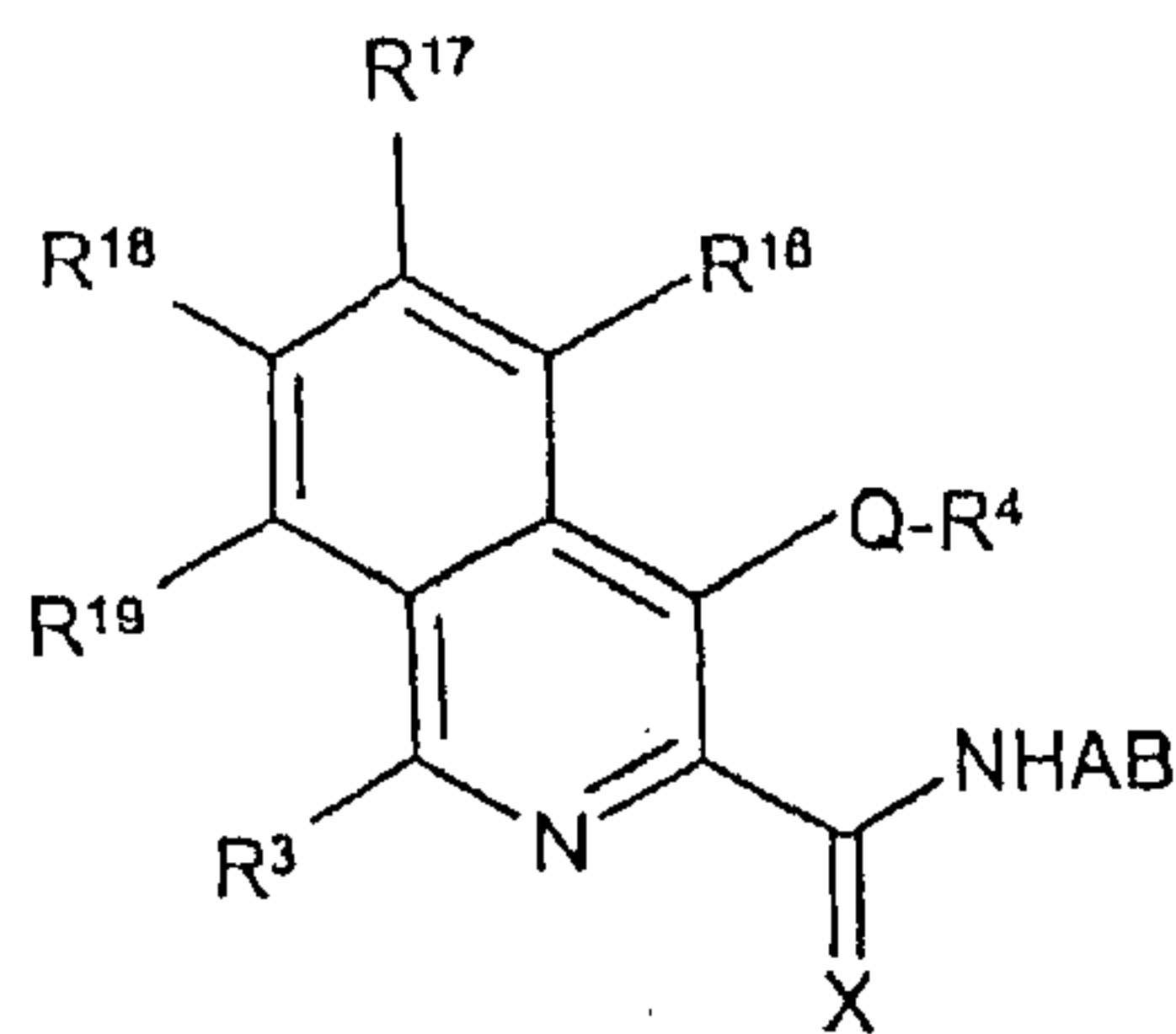
(Ib)
