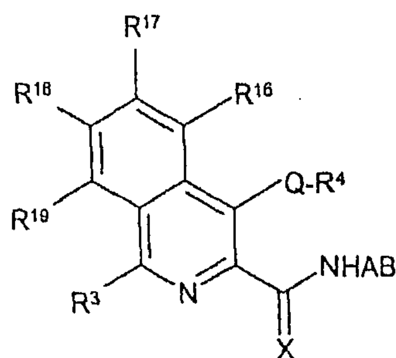
(Ib)
