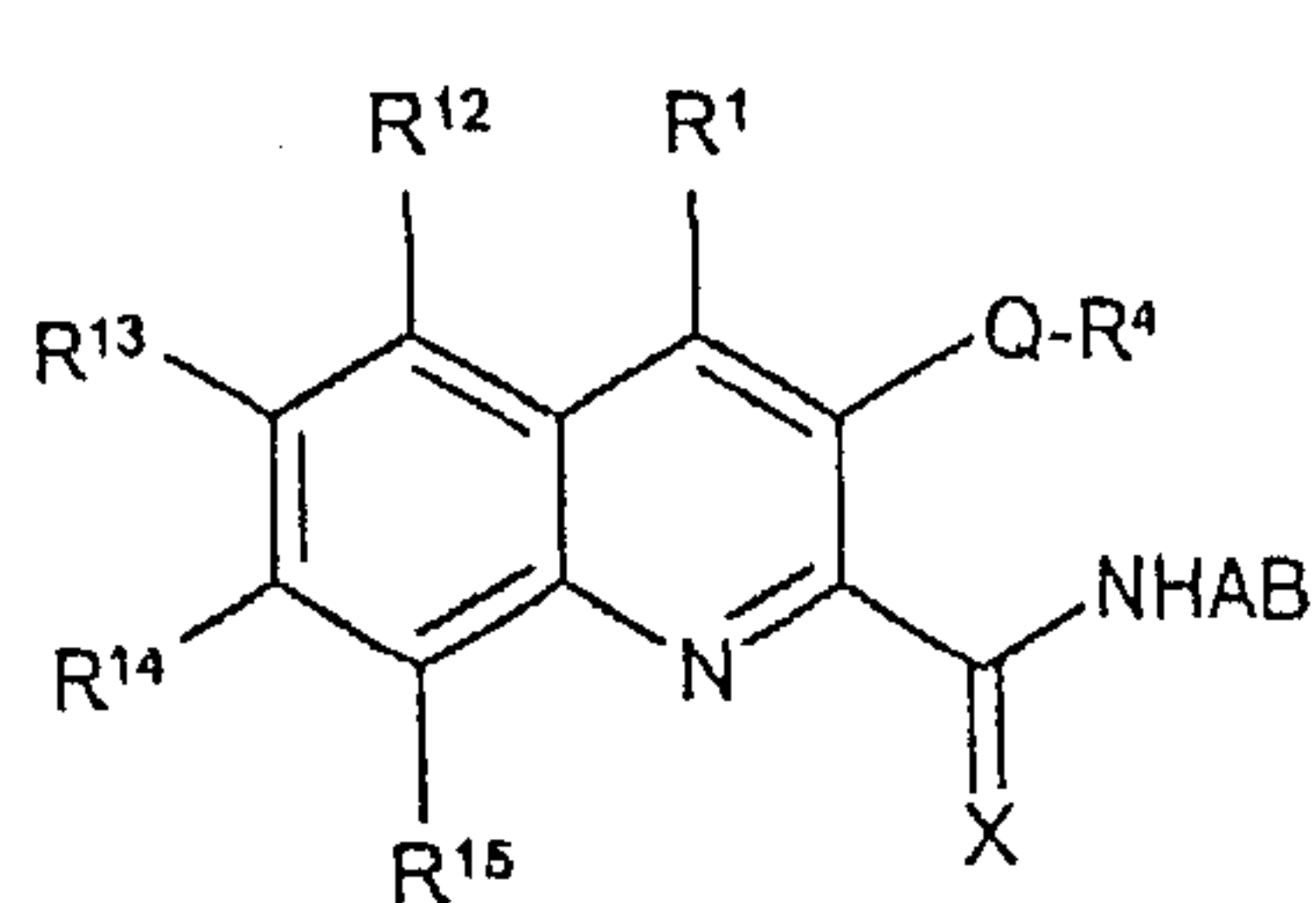
(Ia)
