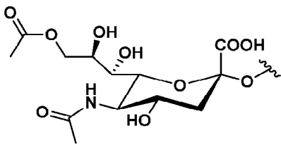
(9AcSA)
