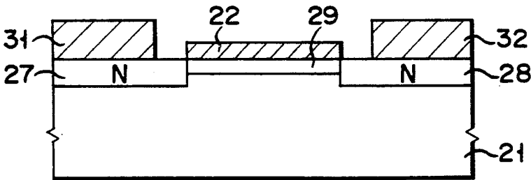
F I G. 2C
