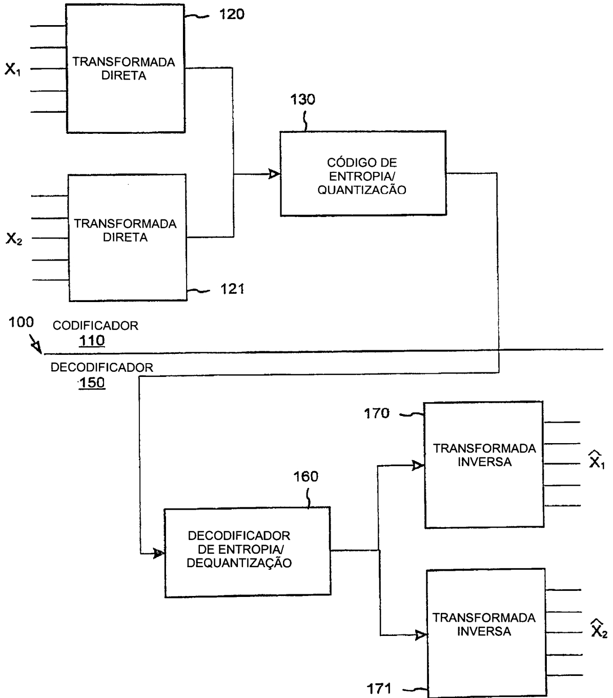
Figura 1 Técnica Anterior
