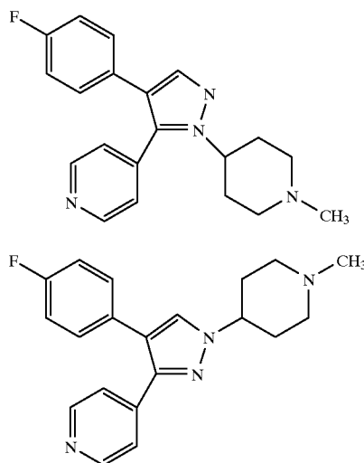
1-methyl-4-[2-[4-(4-fluorophenyl)-3-(4-pyridinyl)-1H-pyrazol-1-yl]]piperidine
