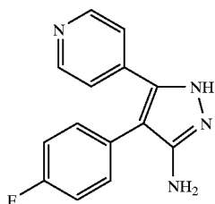
4-(4-fluorophenyl)-5-(4-pyridinyl)-1H-pyrazol-3-amine
