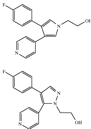
4-(4-fluorophenyl)-3-(4-pyridinyl)-1H-pyrazole-1-ethanol
