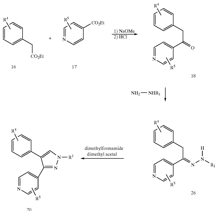
Scheme VI
