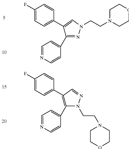
4-[2-[4-(4-fluorophenyl)-3-(4-pyridinyl)-1H-pyrazol-1-yl]ethyl]morpholine
