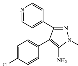
4-(4-chlorophenyl)-1-methyl-3-(4-pyridinyl)-1H- pyrazol-5-amine
