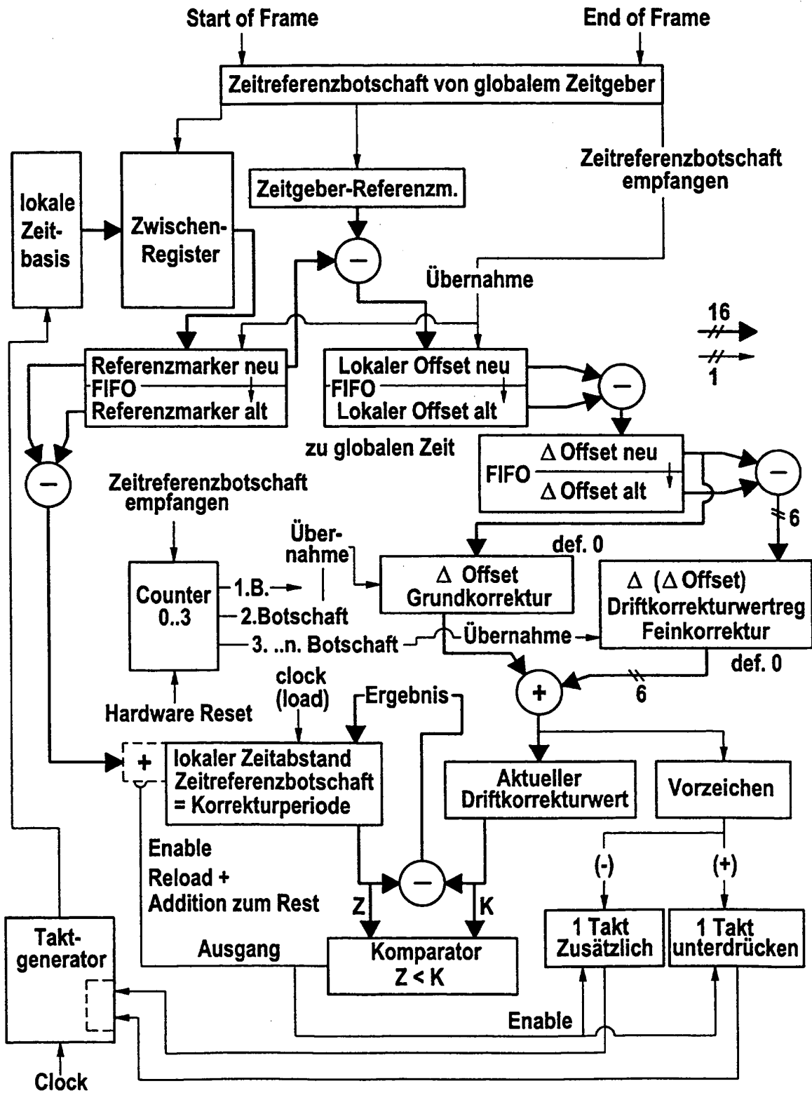
FIG. 6 Driftkorrektur (Blockschaltbild)
