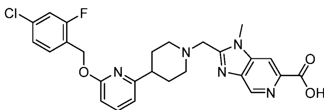
Example 2A-03
