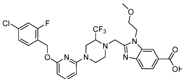
Example 12A-01
