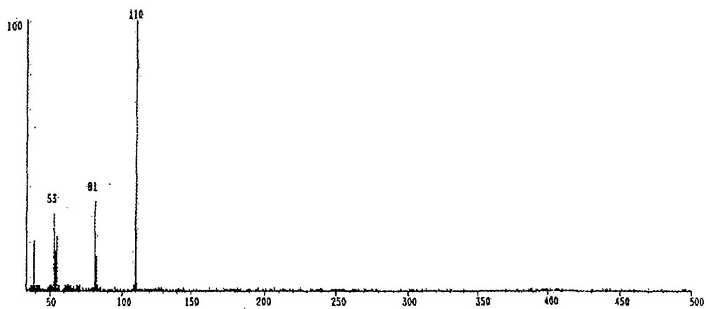
Fig 16. Mass spectrum of the pure cs-oxidant
