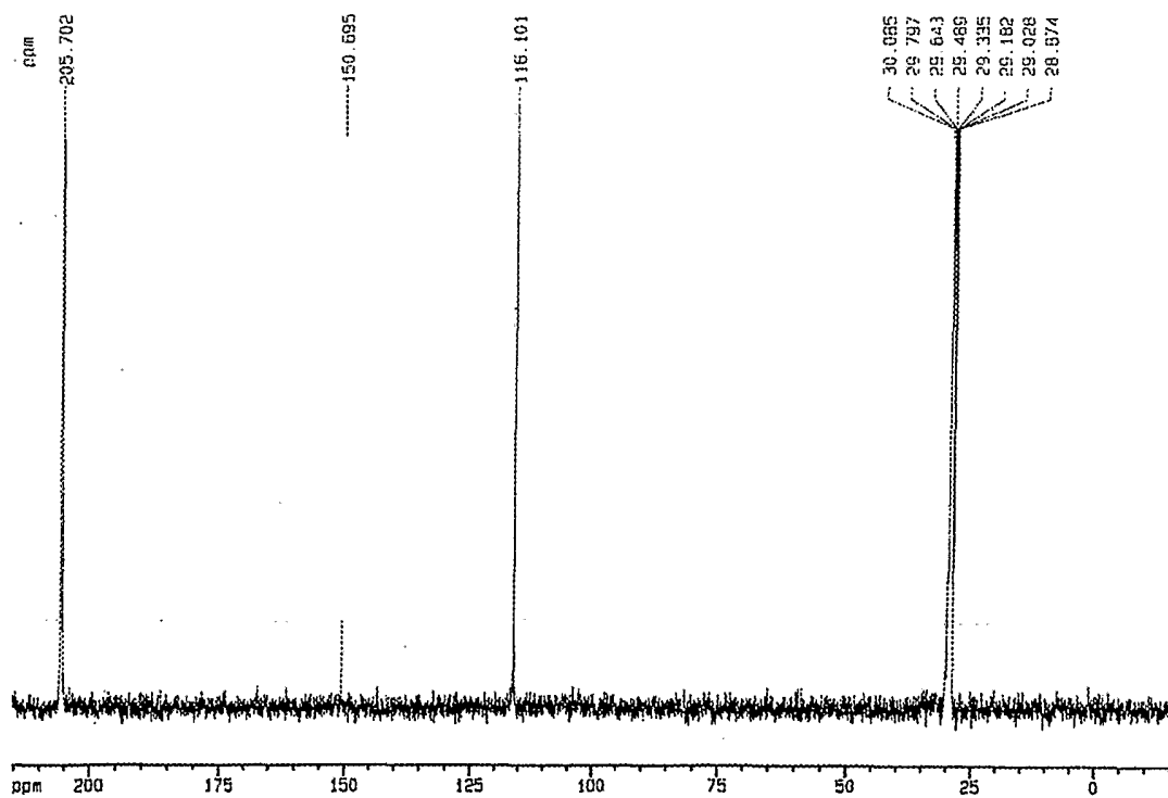
Fig 27. C-NMR spectroscopic profile of the cs-oxidant in CD 3 COCD 3
