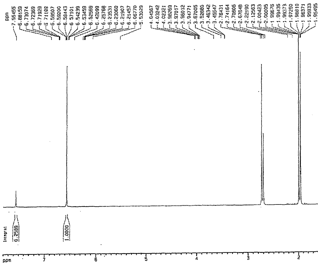
Fig 23. 1 H-NMR spectroscopic profile of the cs-oxidant in CD 3 COCD 3
