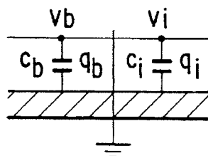
q_b = q_i COLOTRON FIG. 33A
