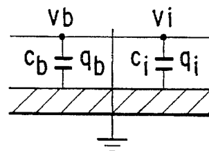
v_b = v_i SCOROTRON FIG. 33B
