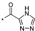
(3.9.10)
