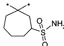
(3.1.18)
