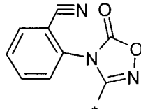
(4.8.38)
