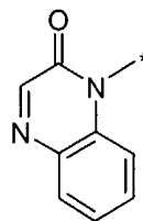
1H-quinoxalin-2-on-1-yl (1.7.15)
