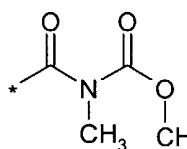
(4.1.3)
