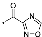
(3.9.15)
