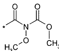
(4.1.5)
