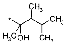
(3.3.6)
