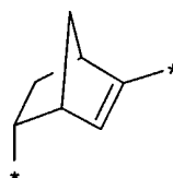
(2.5.29)
