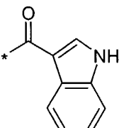
(3.9.27)
