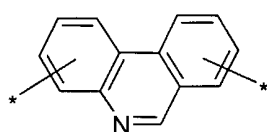
(1.2.19)
