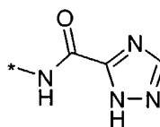
(8.0.3)
