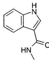
(8.0.127)
