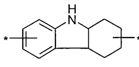
(1.2.14)
