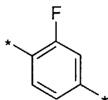
(2.5.1)
