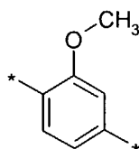
(2.5.6)
