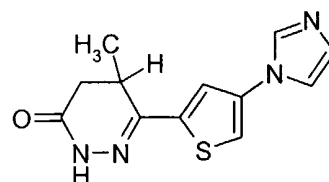
Motapizone
