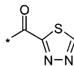
(3.9.17)
