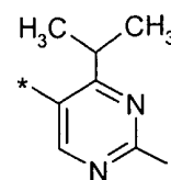
(2.5.16)
