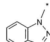
benzotriazolyl (7.5.16)
