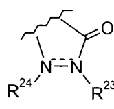
(1.3.13)
