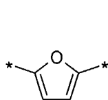
(2.5.33)
