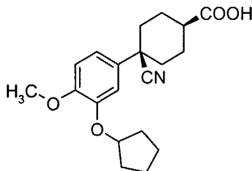
SB-207,499
