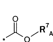
(1.1.1)
