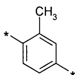
(2.5.41)
