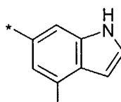
(2.5.35)
