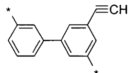
(2.6.12)
