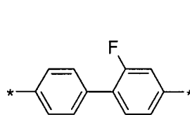
(2.6.8)
