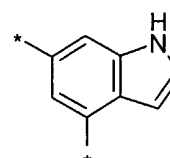
(2.5.35)
