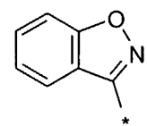
benzisoxazolyl
