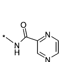
(8.0.125)
