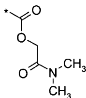
(3.5.12)
