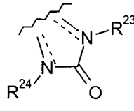
(1.3.14)
