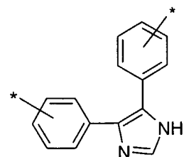
(1.2.10)
