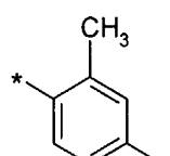
(2.5.41)
