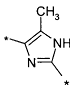
(2.5.18)
