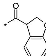
(3.9.29)
