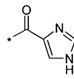
(3.9.13)
