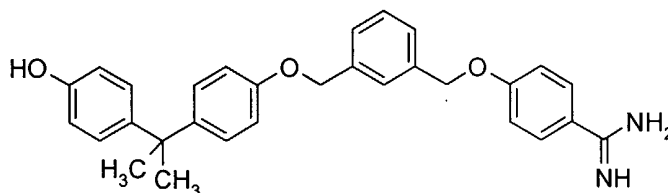
BIIL 284/260
