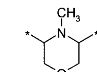
(2.5.44)
