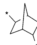
(2.5.28)
