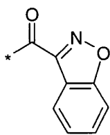
(3.9.36)
