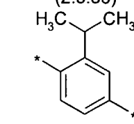
(2.5.40)
