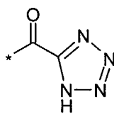
(3.9.11)
