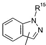
1H-indazolyl
