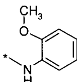
(8.0.134)
