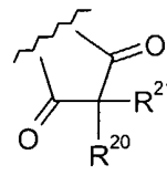
(1.3.9)
