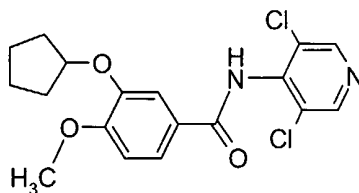
Piclamilast (RP-73,401)
