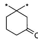
(3.1.15)
