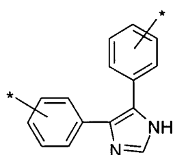
(1.2.10)
