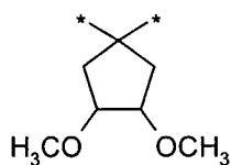
(3.1.12)
