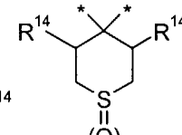
(1.5.11)
