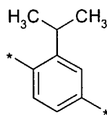
(3.0.64)
