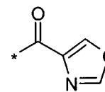
(3.9.19)
