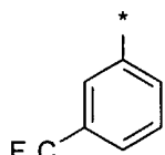
(2.0.9)
