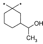
(3.1.34)
