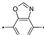
(2.5.46)
