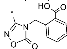
(4.8.36)
