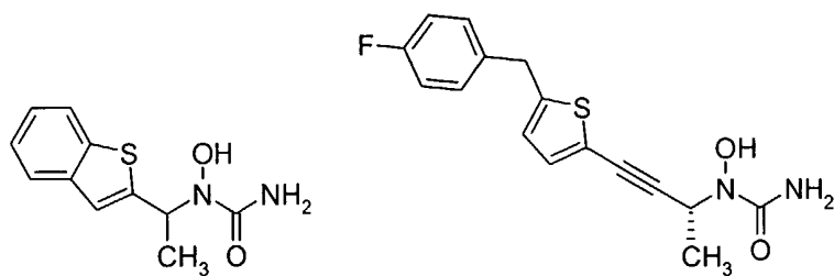
Zileuton
