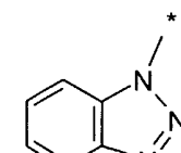
benzotriazolyl
