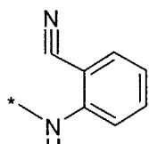
(8.0.135)
