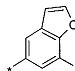
(3.0.69)
