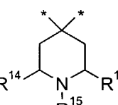
(1.5.10)
