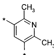
(2.5.15)
