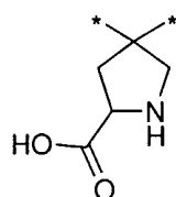
(3.1.28)
