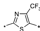
(2.5.20)
