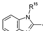
benzimidazolyl (7.5.11)
