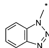
benzotriazolyl
