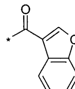
(3.9.28)
