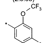
(2.5.39)
