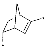
(2.5.29)
