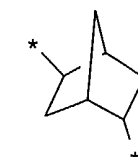
(2.5.28)
