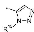
1,2,3-triazol-5-yl (1.4.4)
