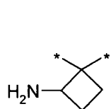
(3.1.6)
