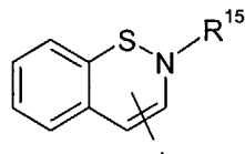
2H-1,2-benzothiazinyl
