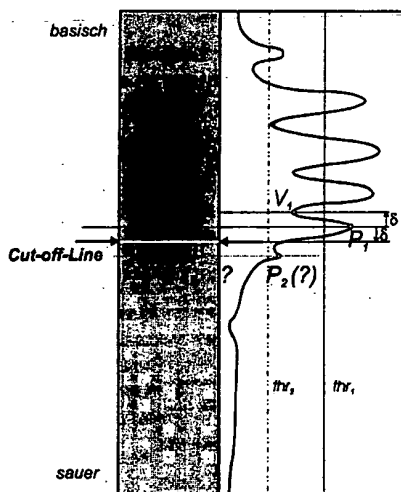
Abbildung 2: Konventionelle Methode der Cut-off-Line Ermittlung
