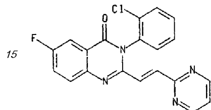
Сполука 47
