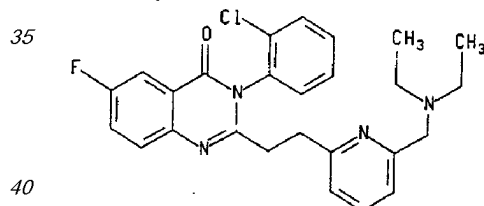
Сполука 49
