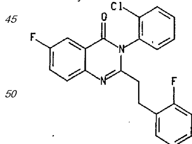
Сполука 50
