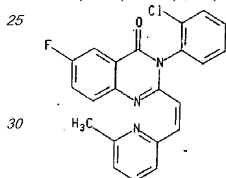
Сполука 49
