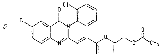
Сполука 46
