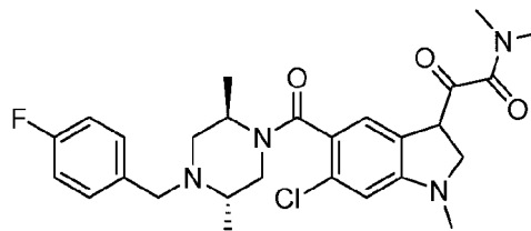
SCIO 469
