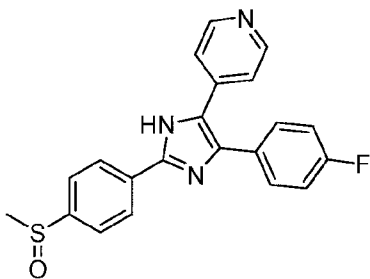
SB-203580
