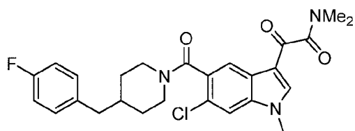
SX 011
