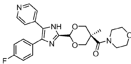
RPR-200765A
