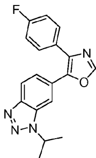
4-(4-fluorophenyl)-5-(1-isopropyl-1H-benzo[d][1,2,3]triazol-6-yl)oxazole
