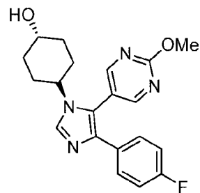
SB 239063
