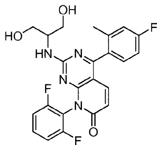
SB-681323
