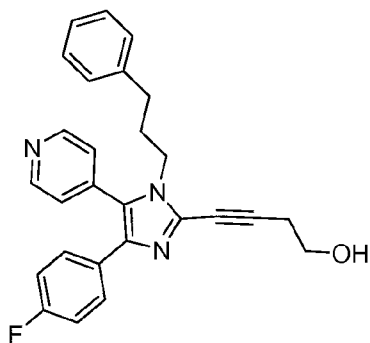
RWJ 67657
