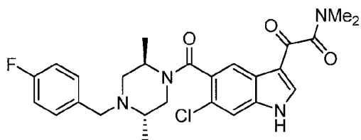
SD 282
