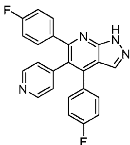
Org 48762-0
