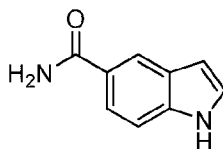
SD 169
