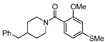
JX 401
