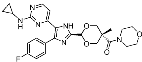
RPR-203494
