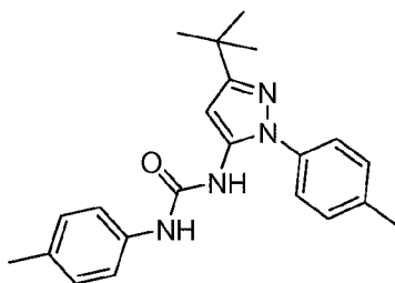
1-(3-tert-butyl-1-p-tolyl-1H-pyrazol-5-yl)-3-p-tolylurea
