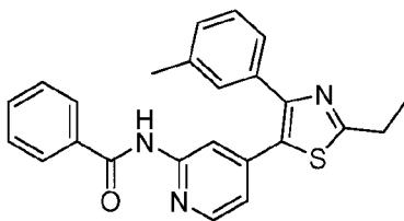
TAK-715
