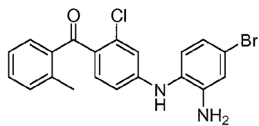
EO 1428
