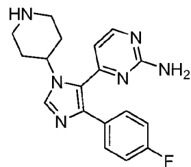
SB-200025
