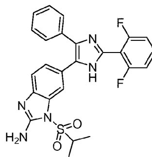
6-(2-(2,6-difluorophenyl)-4-phenyl-1H-imidazol-5-yl)-1-(isopropylsulfonyl)-1H-benzo[d]imidazol-2-amine
