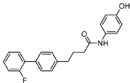
CMPD1
