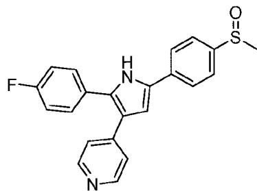
L-167307
