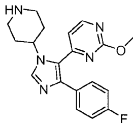
SB-242235
