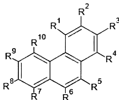
(VII)
