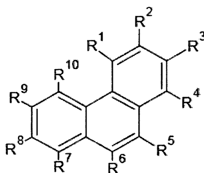
(II)
