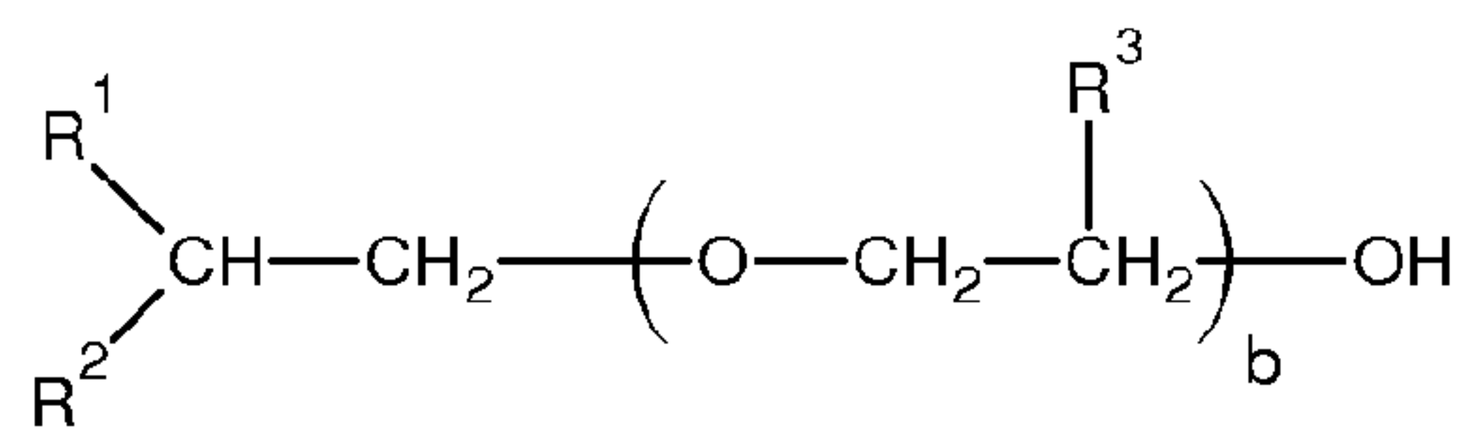
Formula I:
