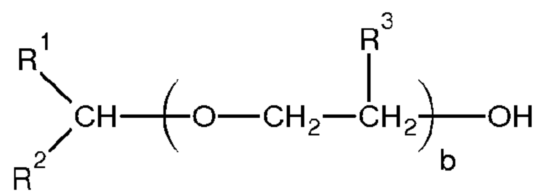
Formula II:
