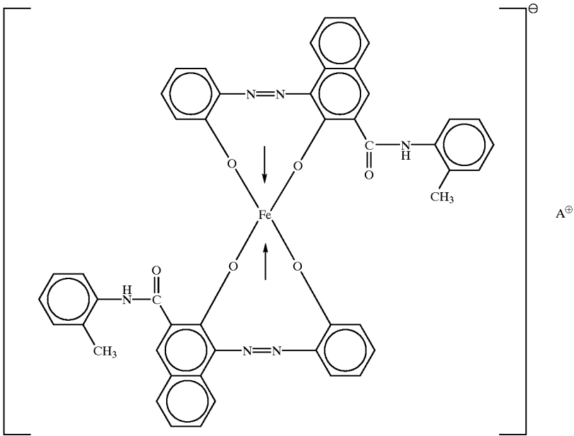
Azo ion complex (6)
