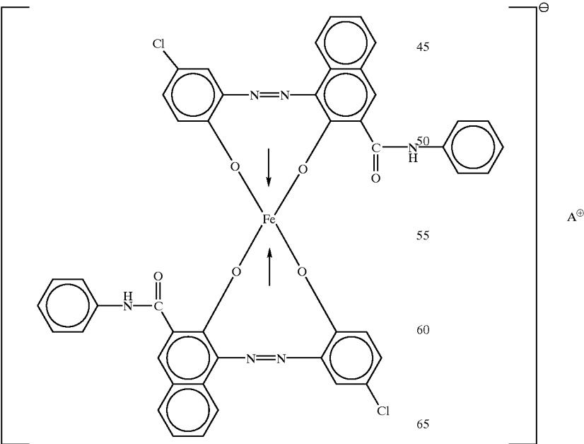
Azo ion complex (1)
