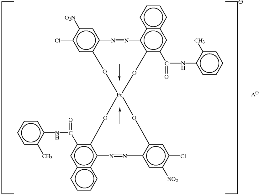
Azo ion complex (5)
