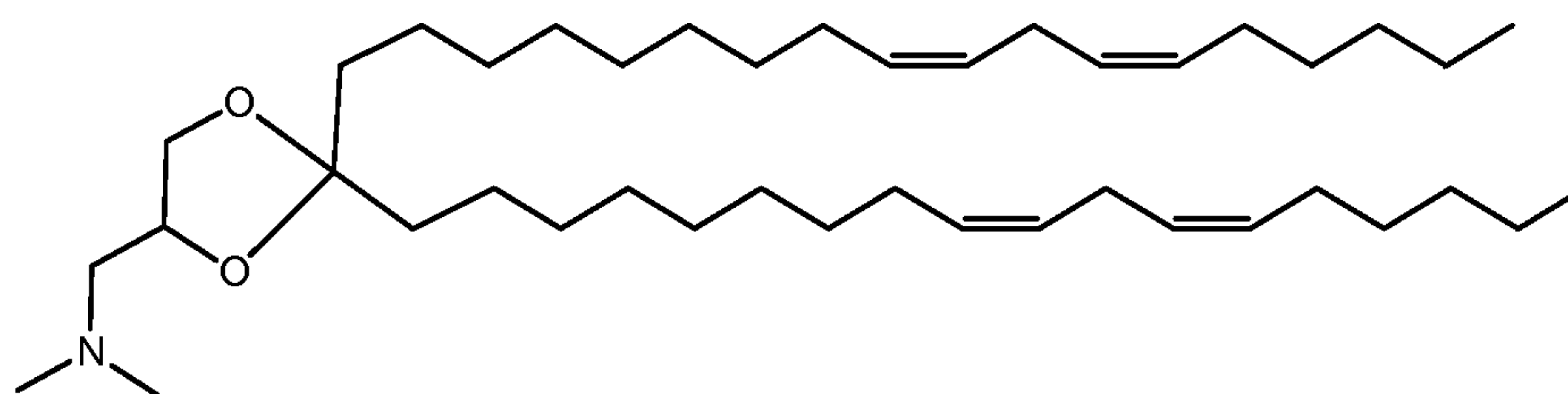
DLin-K-DMA.
