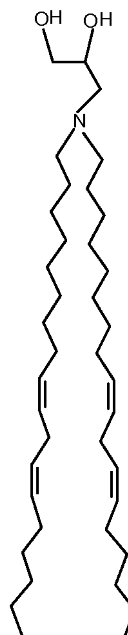
DLinAP 3-(Dilinoyleylamino)-1,2-propanediol
