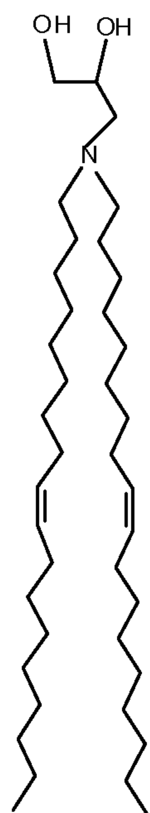
DOAP 3-(Dioleylamino)-1,2-propanediol
