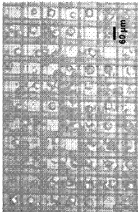
Lysozyme
