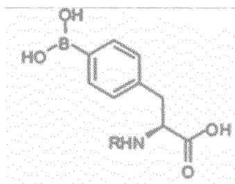
formule (II) ;
