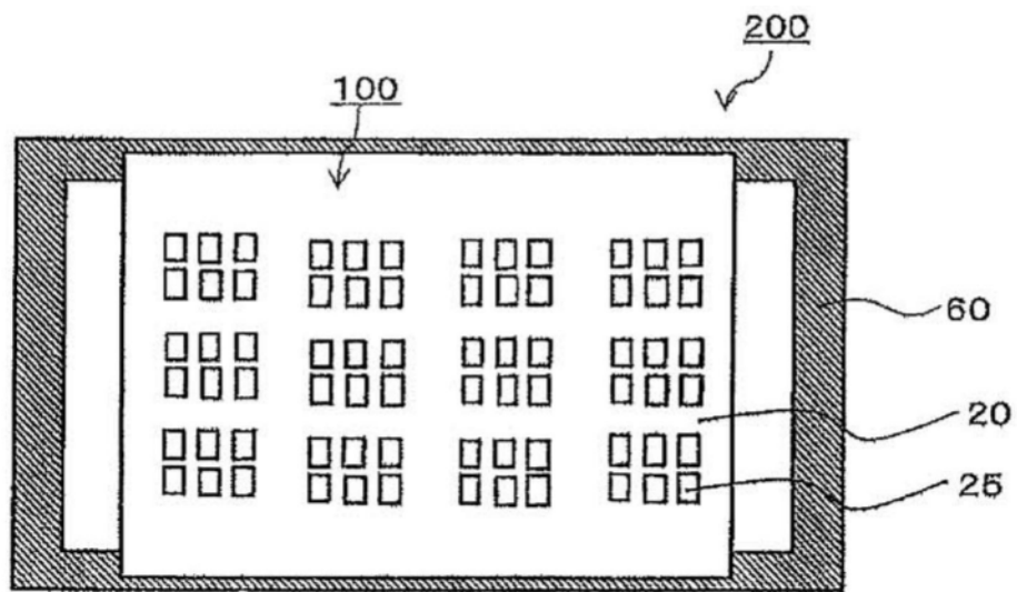
从树脂掩模侧观察的图
