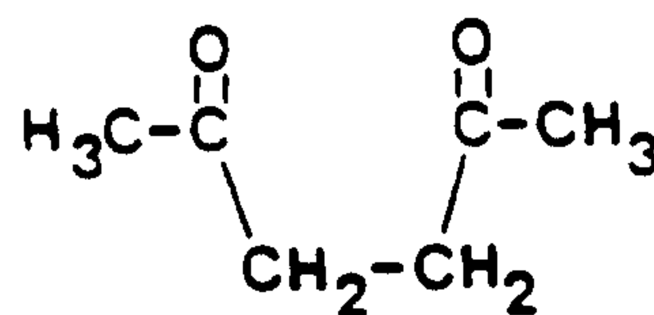
2,5-hexanedione
