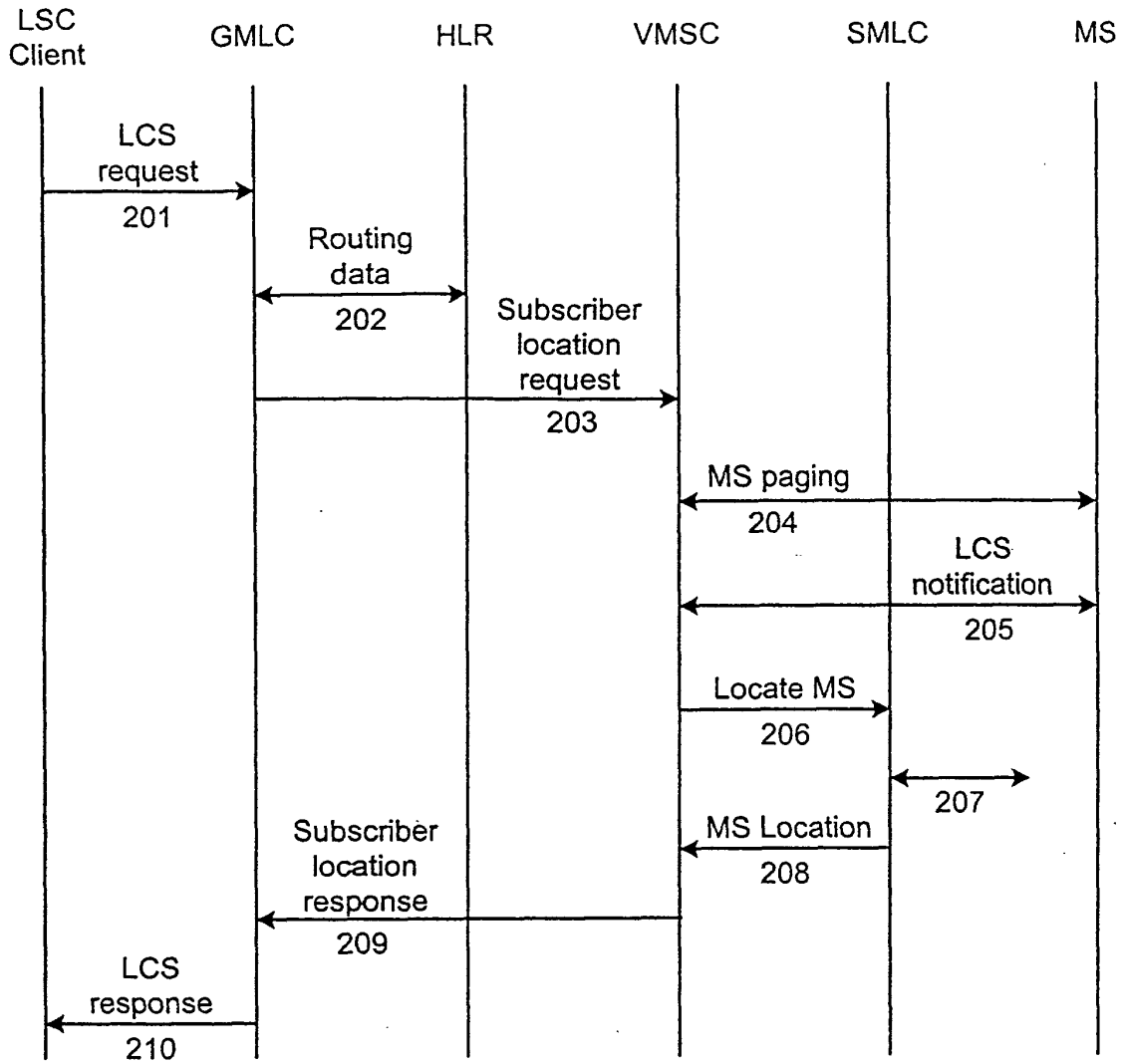
FIG. 2 PRIORT ART
