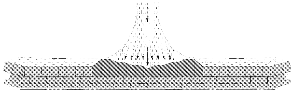
Fig. 1b Înzidire căptușeală Oala Torpedo cu zona de impact fără bazin/baie de protecție (schema) – exemplu de uzura a zidăriei de impact în cazul lipsei bazinului de formare a băii de protecție conform invenției.
