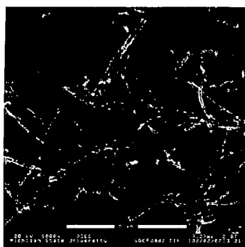
B: VGCF (Scale Bar = 5um)
