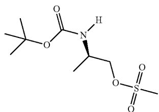
A. (R)-2-((tert-Butoxycarbonyl)amino)propyl methanesulfonate
