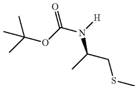
B. (R)-tert-Butyl (1-(methylthio)propan-2-yl)carbamate
