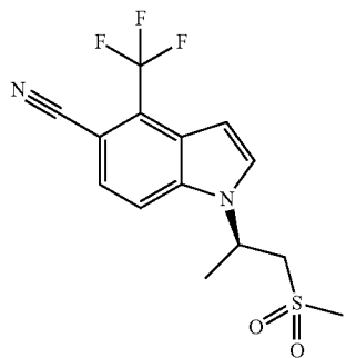
E. (R)-1-(1-(Methylsulfonyl)propan-2-yl)-4-(trifluoromethyl)-1H-indole-5-carbonitrile
