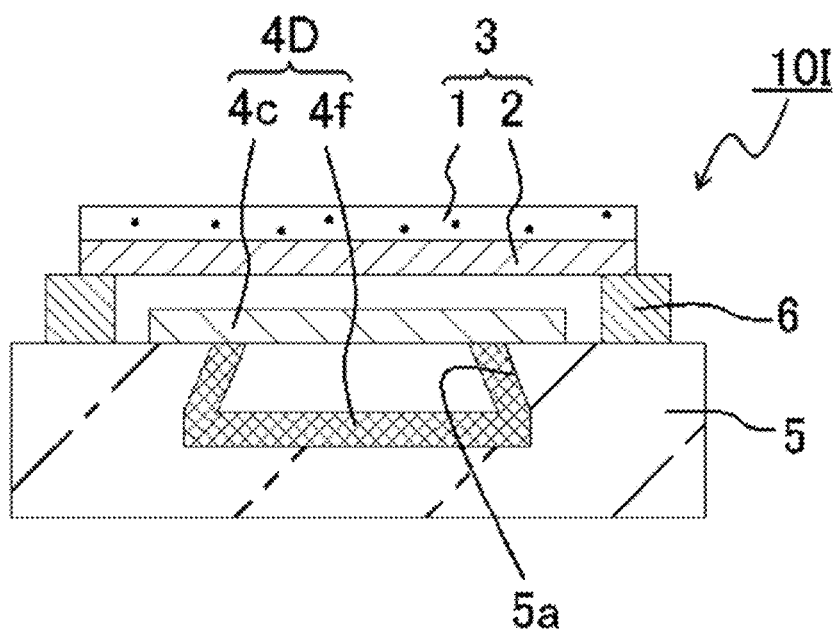
FIG. 1I
