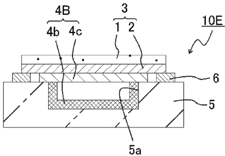
FIG.1E
