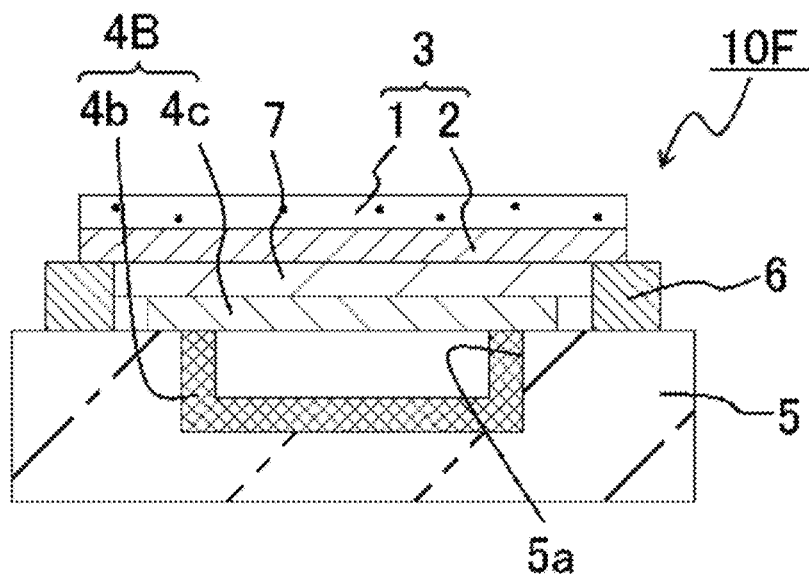
FIG.1F
