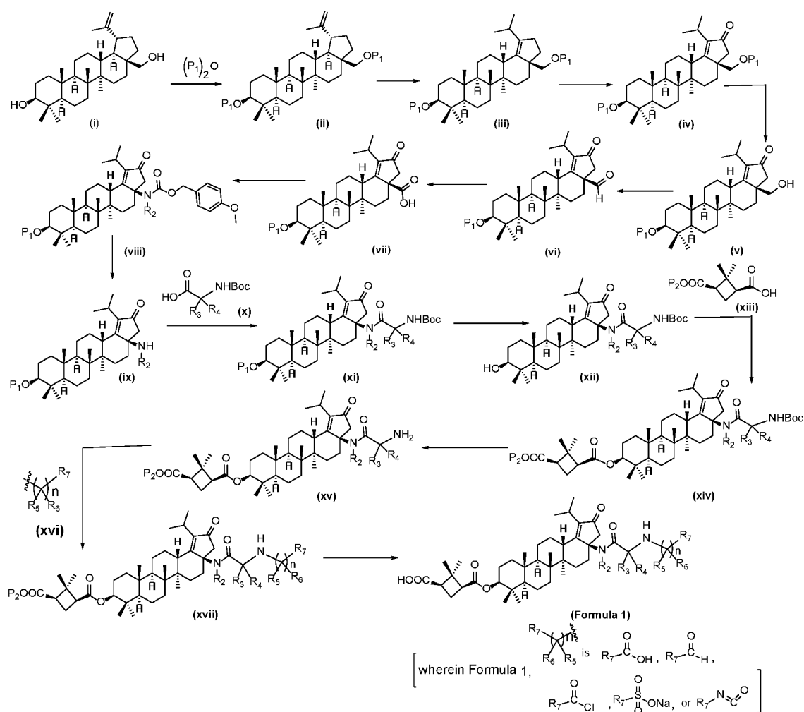
Scheme-1
