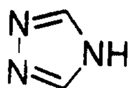
triazole (triazolyl)
