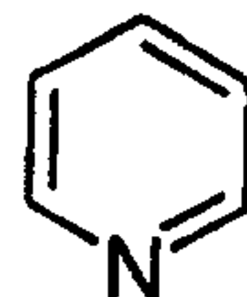
pyridine (pyridinyl)
