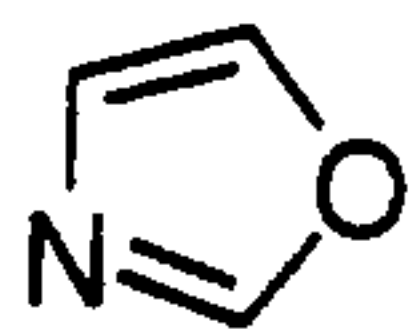
oxazole (oxazolyl)
