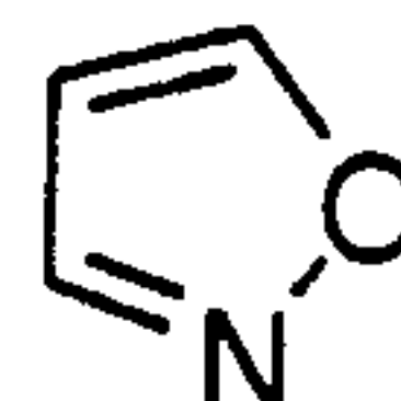
isoxazole (isoxazolyl)
