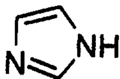
imidazole (imidazolyl)
