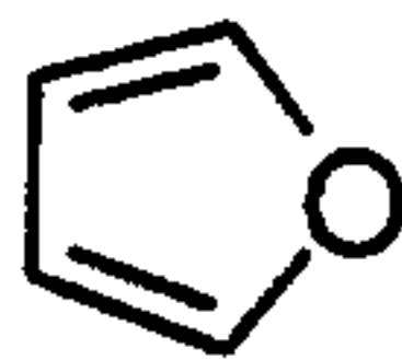
furan (furyl)
