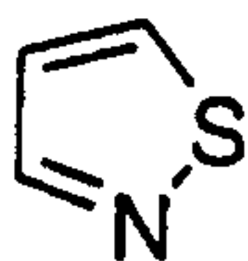
isothiazole (isothiazolyl)
