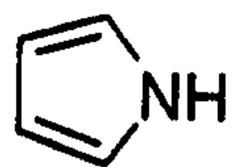
pyrrole (pyrrolyl)
