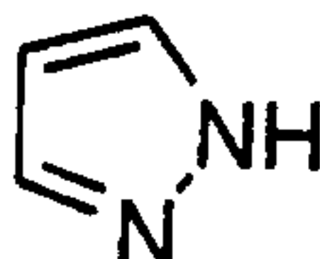
pyrazole (pyrazolyl)
