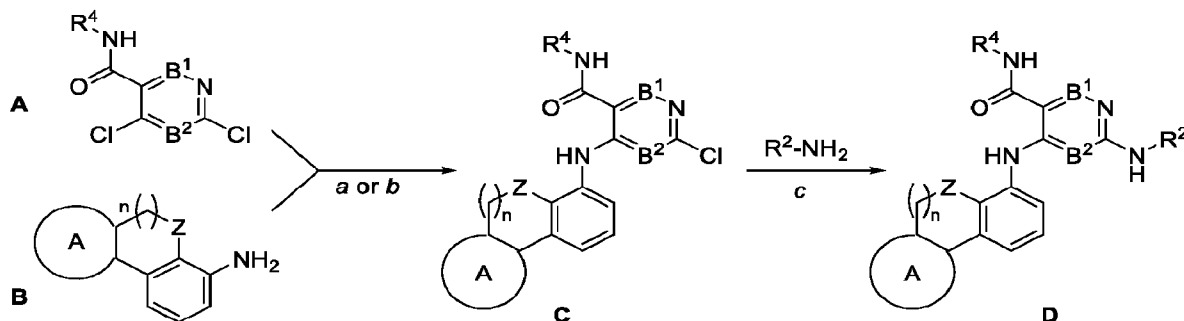
Scheme A:
