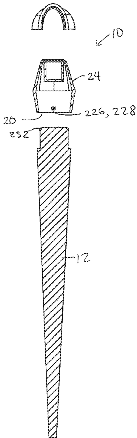
Fig. 15A Section A-A
