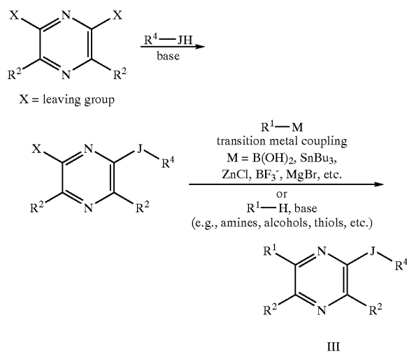
Scheme 3.a
