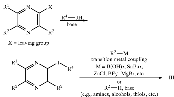
Scheme 3.b
