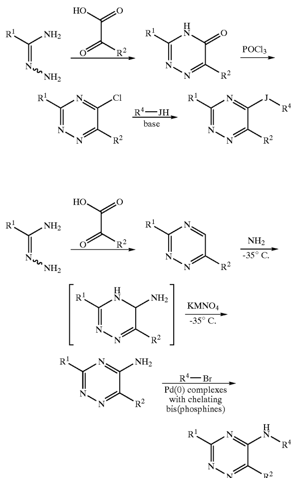
Scheme 2.a
