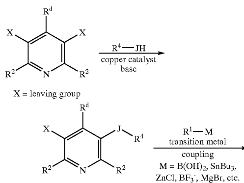
Scheme 4.a
