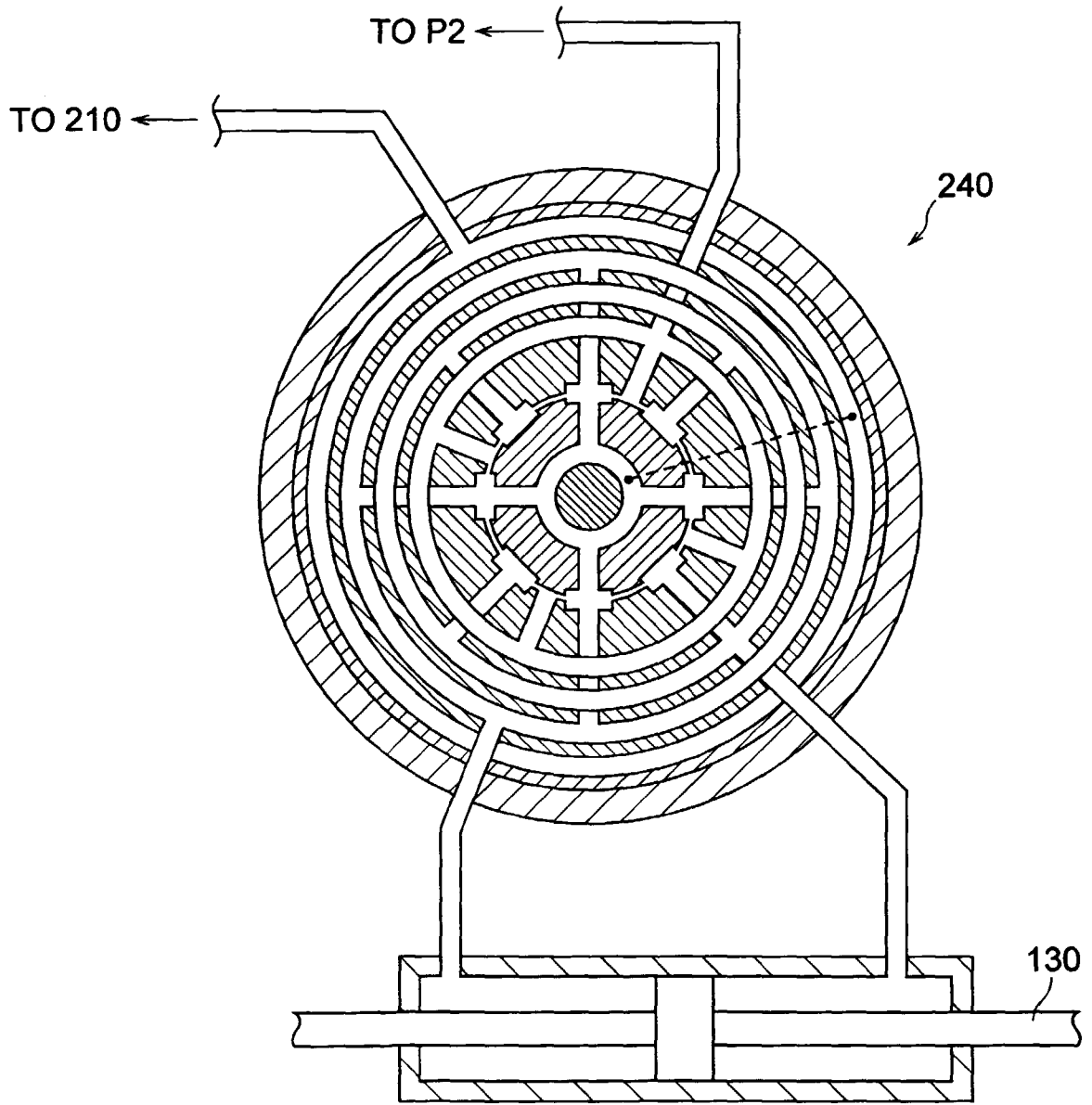
A-A SECTION
