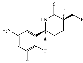
(3S,6S)-6-(5-amino-2,3-difluorophenyl)-3-fluoro-3-(fluoromethyl)-6-methylpiperidine-2-thione
