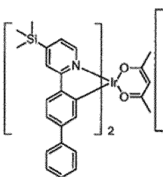
[Formule chimique Q-30]
