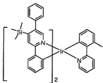
[Formule chimique P-19]
