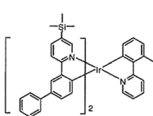
[Formule chimique P-20]
