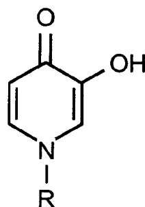
Pyridine-4-ones
