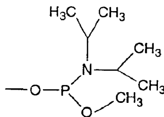
N,N-diisopropylamino-methoxyphosphine
