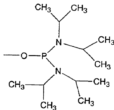
Bis(N,N-diisopropylamino)- phosphine
