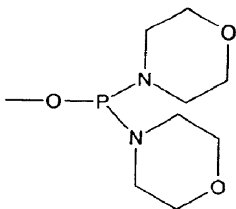
Bis morpholino-phosphine
